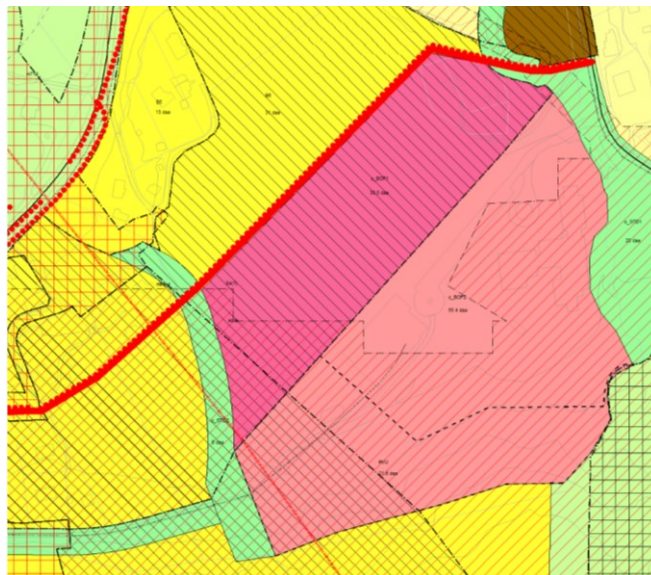
Figur 5-3 Fremtidig samleveg, Sa(1), ved Sundvollen oppvekstsenter
