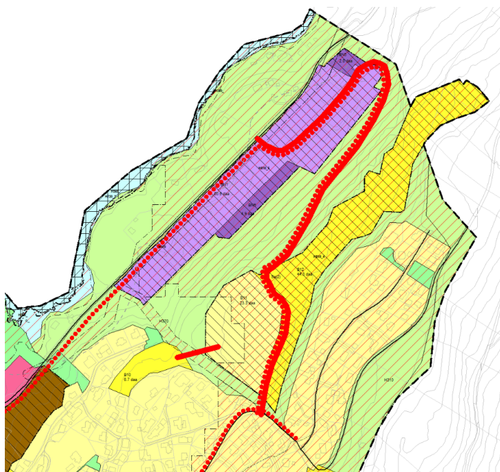
Figur 5-2 Fremtidig veilinje Sa(2) for ny Trøgslevei
